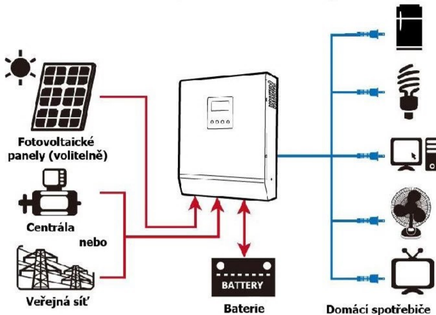
Obrázek 1: hybridní systém
